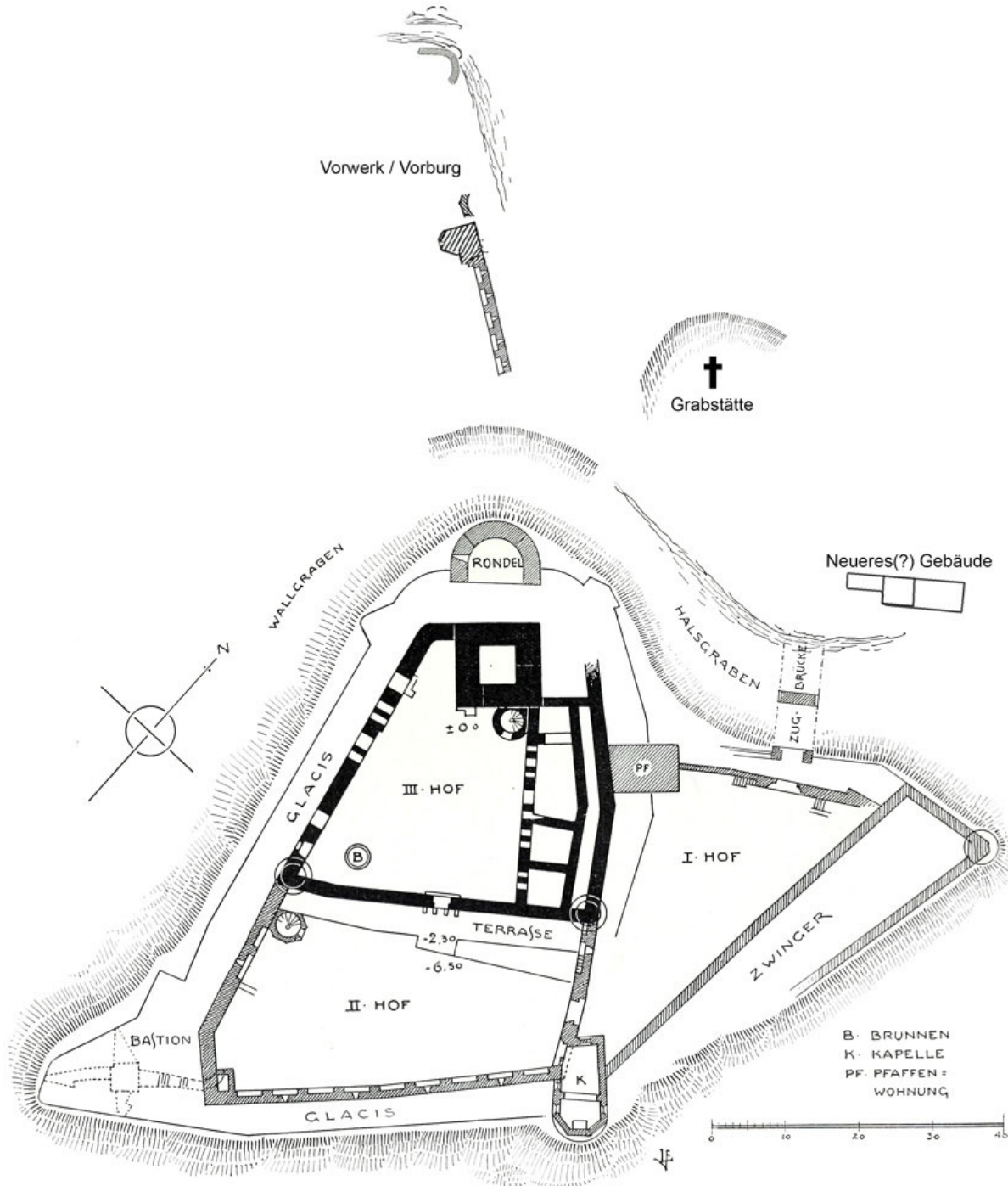
Sauerburg, Sauerthal. Grundriss nach Aufnahme von Prof. Löhr, erweitert durch A. Winkler.
