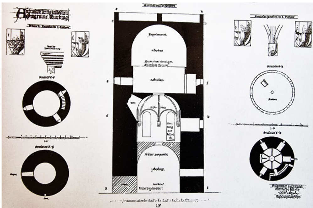
Quelle: osse, Michael - Keck und fest, mit senkrechten Mauertürmen ... wie eine Krone | Regensburg, 2008 | S.127 Nürnberg Wohnturm. Schnitt, Grundrisse und Details (Karl Meyer, 1901).
